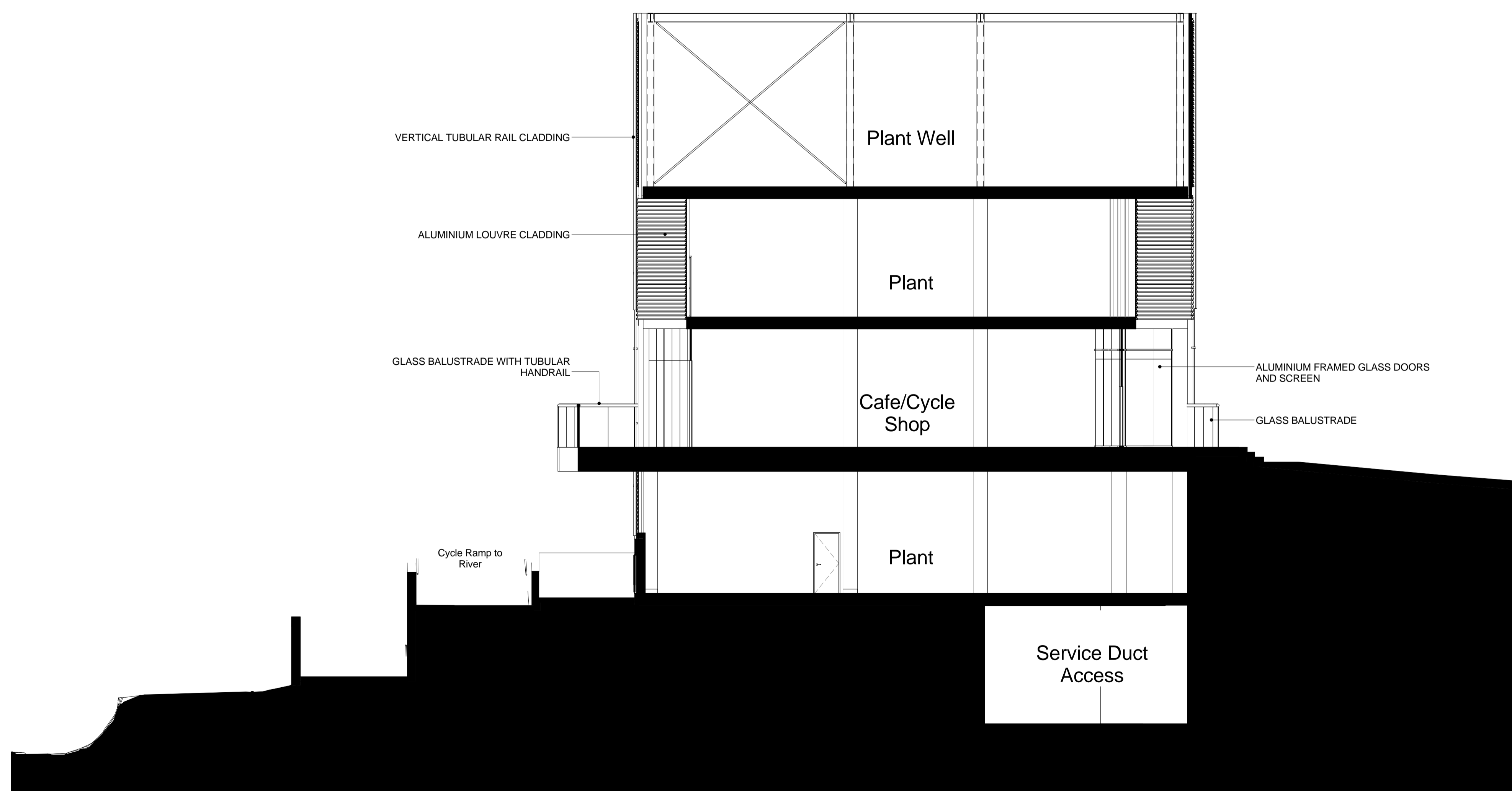
1 GA Cross Section 2' 2 1 : 100
