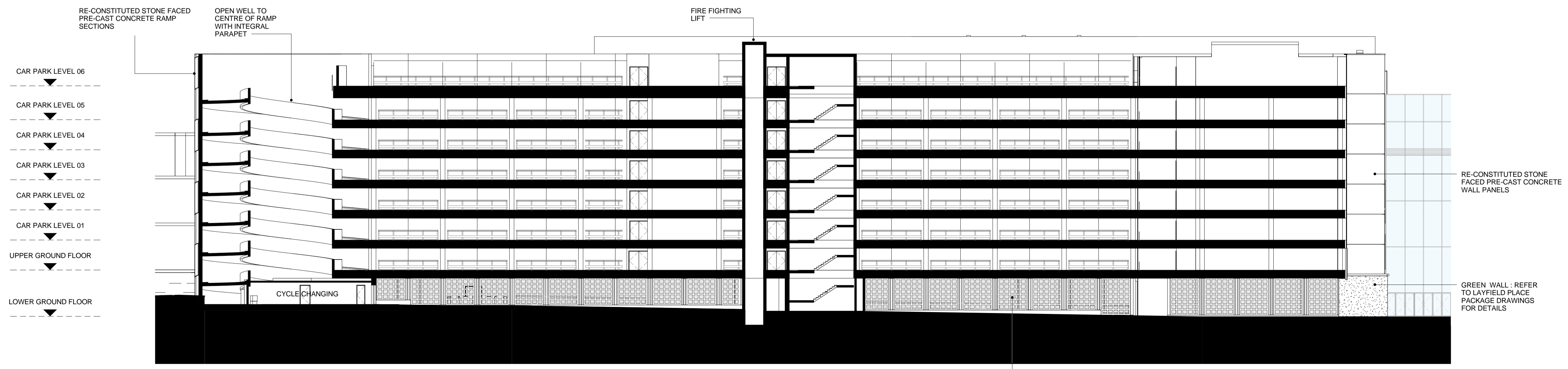
2 GA Long Section - B-B 1 : 250
