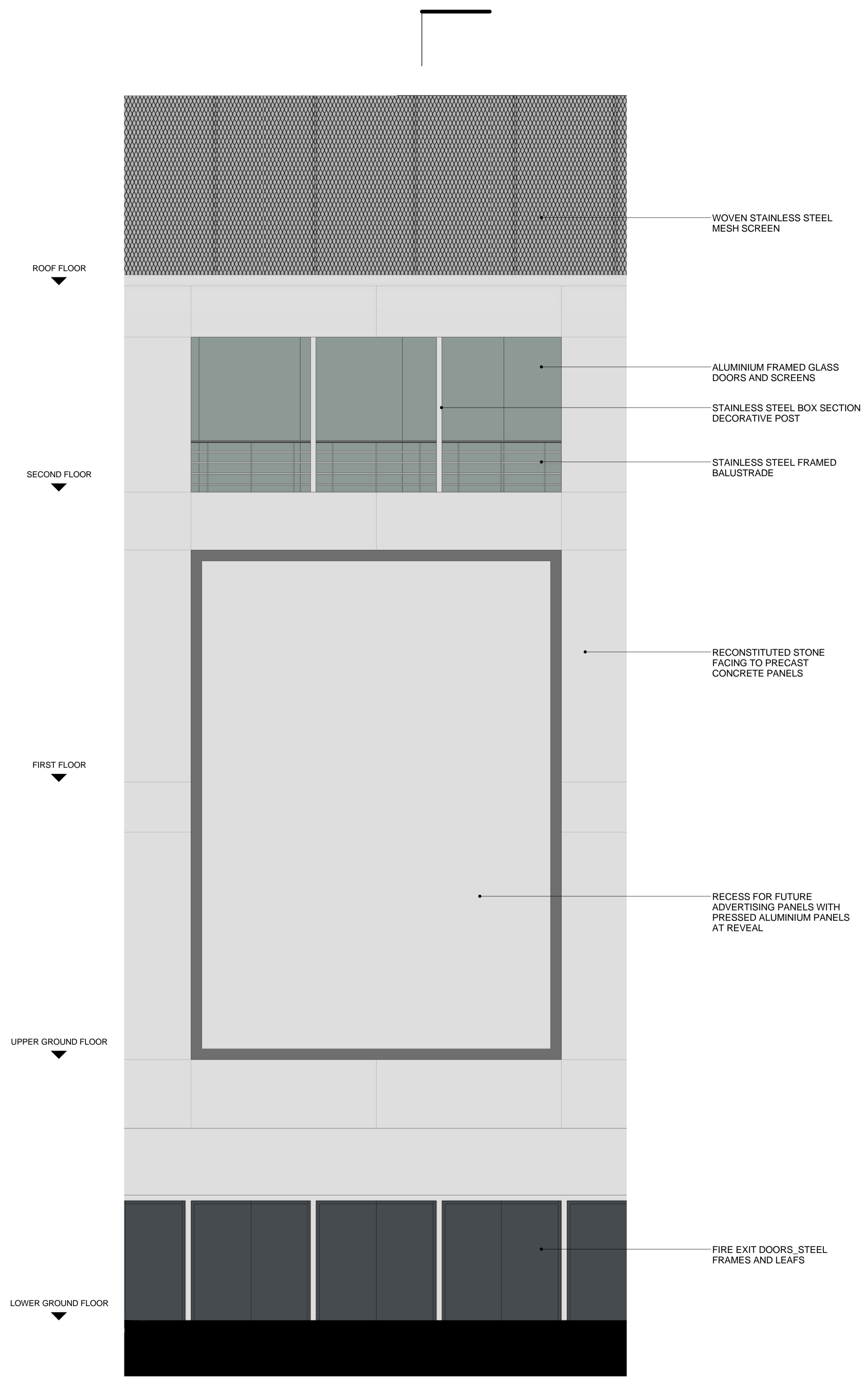
1 ELEVATION 1 : 50
